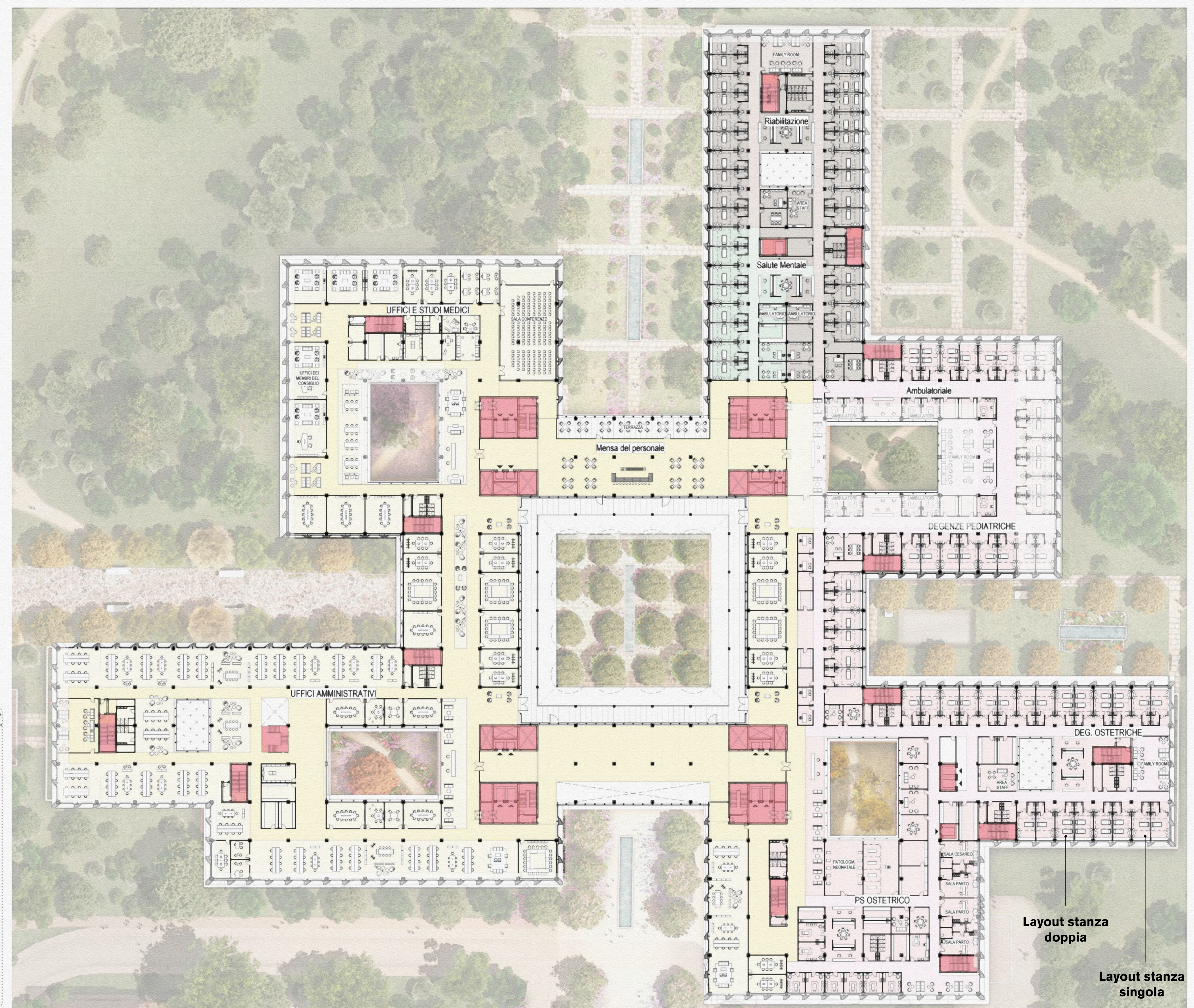
Diagramma Operativo - Percorsi Pianta Piano Primo - 1:400
