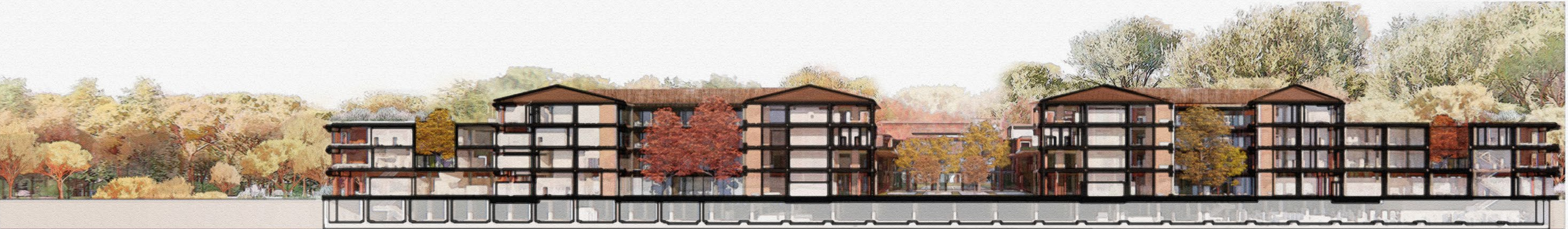
Sezione 1:40C
